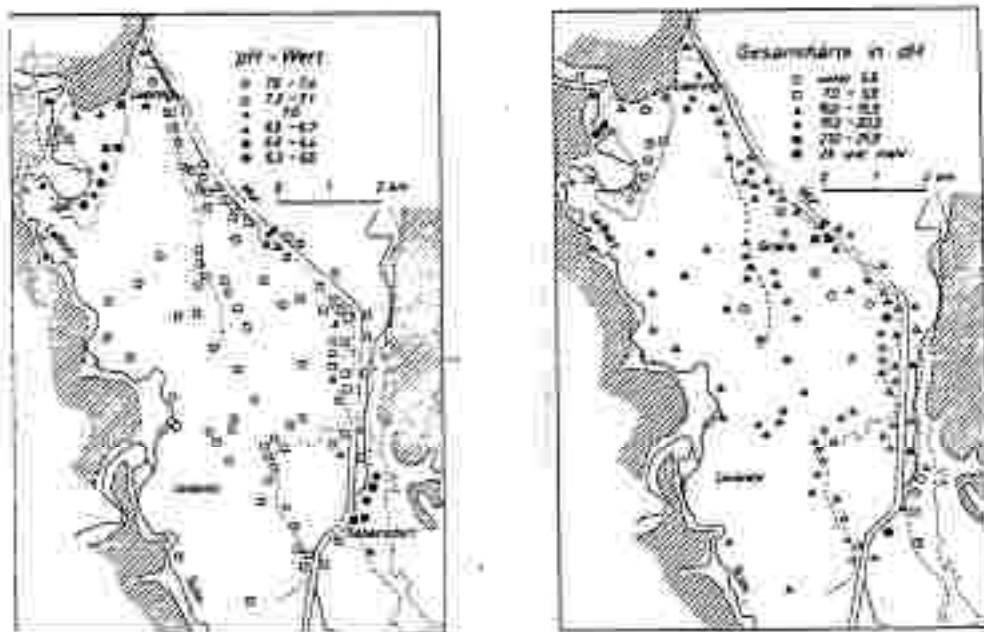
Der pH-Wert von Wässern im Leibnitzerfeld im Juli 1965.
