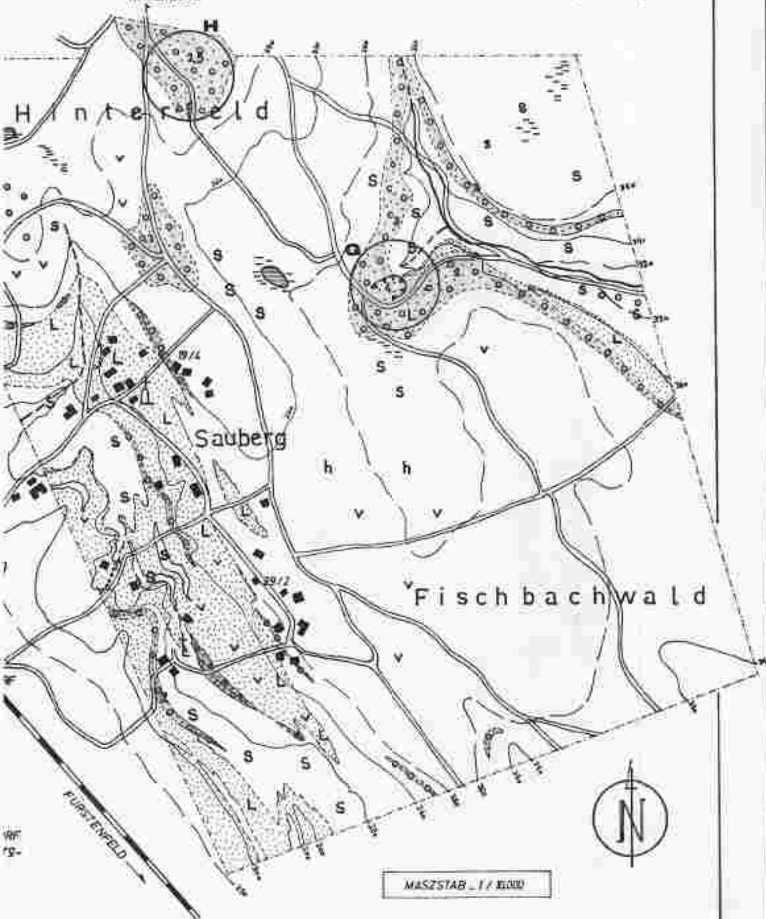
GEOLOGISCHE KARTE DES GEBIETES SÜDLICH VON WAGERBERG ( Oststeiermark )
