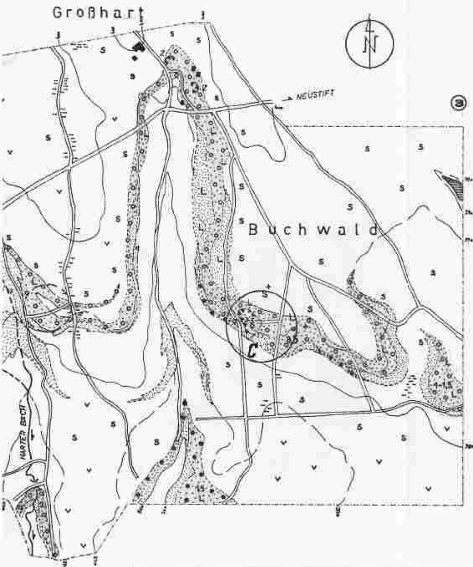
GEOLOGISCHE KARTE DES GEBIETES SÜDLICH VON GROSSHART ( Oststeiermark )
