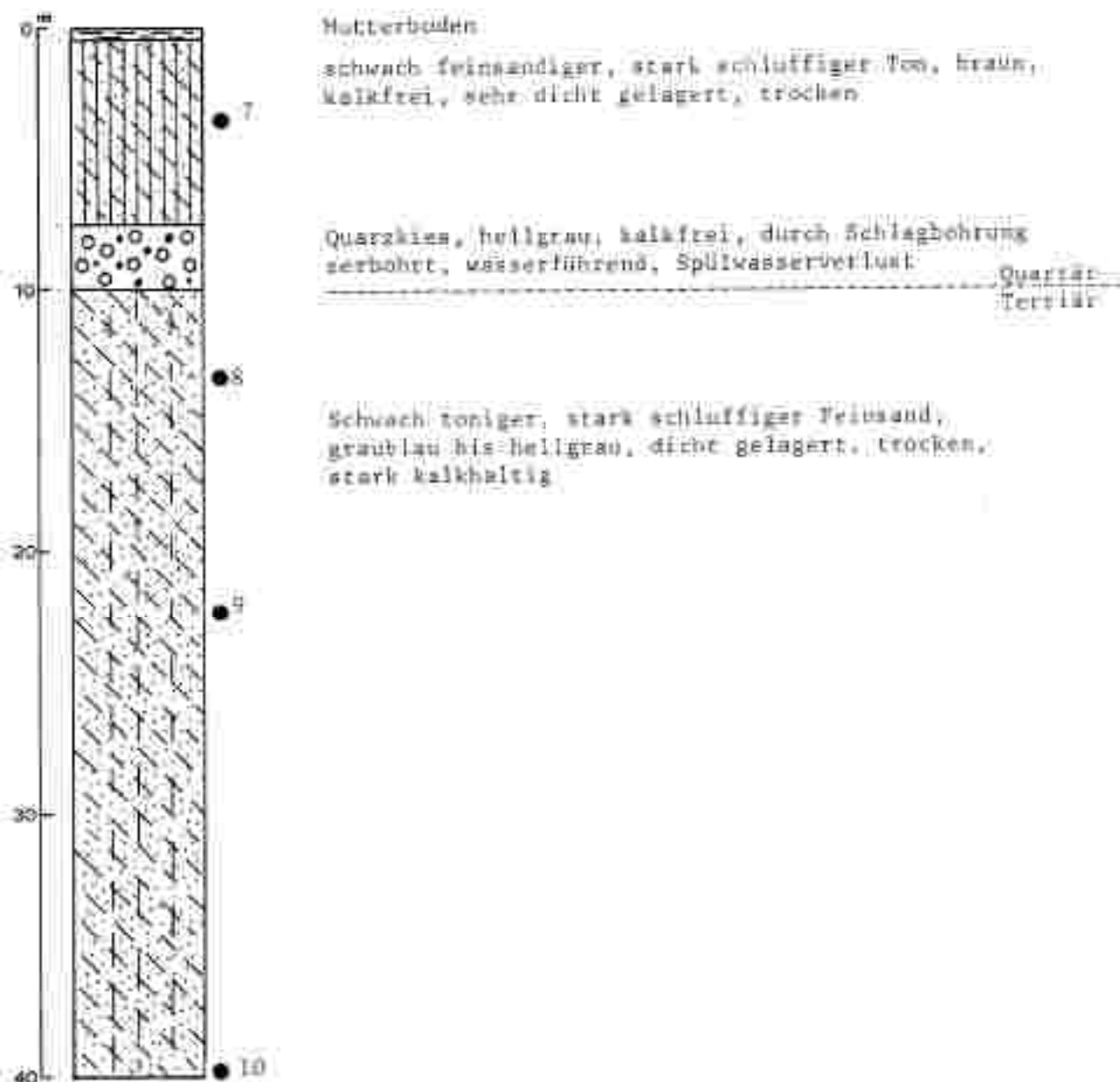
Fig. 7: Bohrprofil der Sonde 2 in Halbenrain (H 2) Darstellung und Benennung nach DIN 4033
