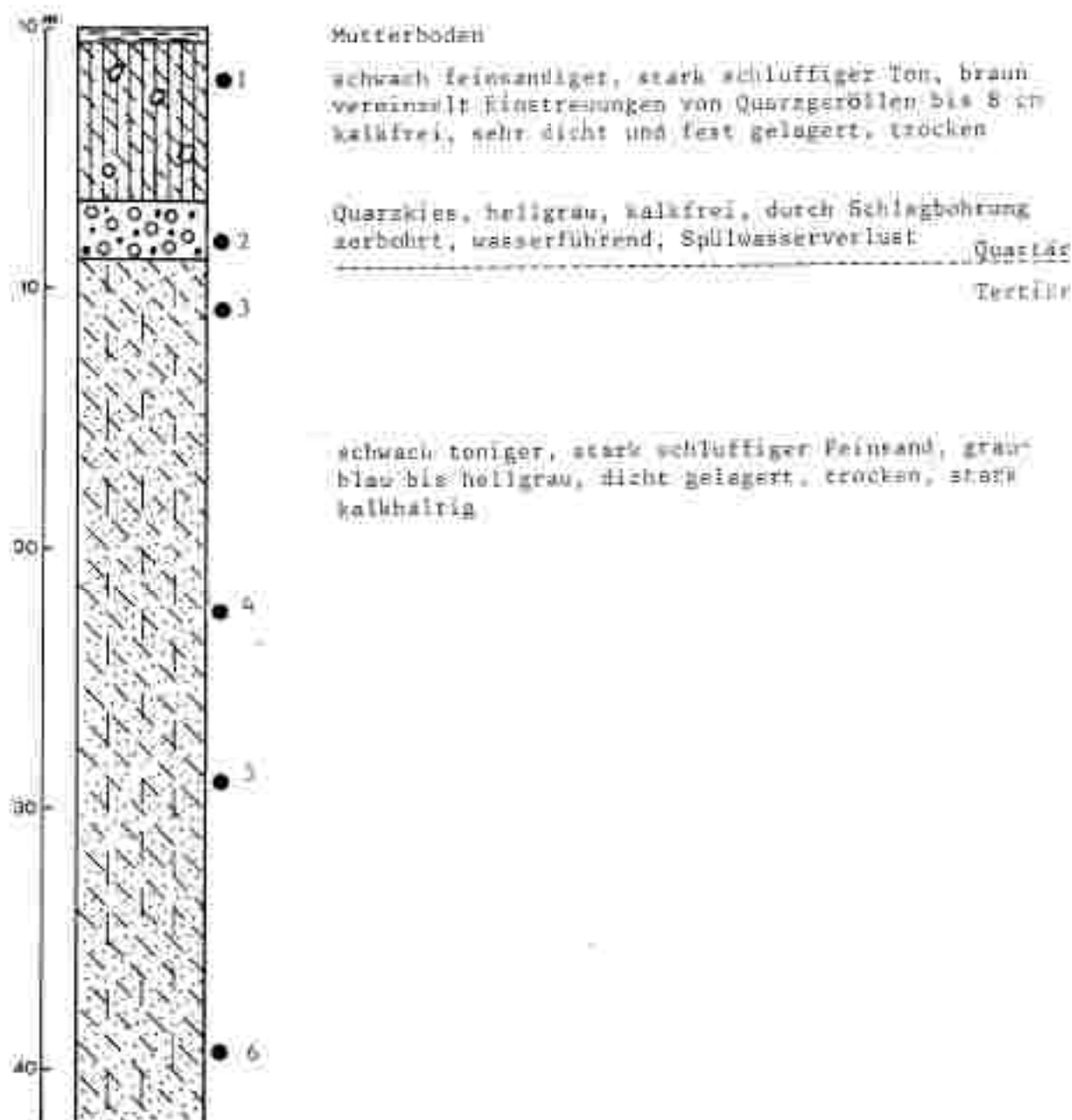
Fig. 6: Bohrprofil der Sonde in Unterputzle (S 1) Darstellung und Benennung nach DIN 4033
