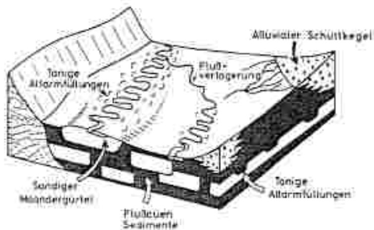
Abb. 3: Vereinfachtes Schema zum internen Aufbau der Flußablagungen der Kies/Sand/Schluff-Wechselfolge
