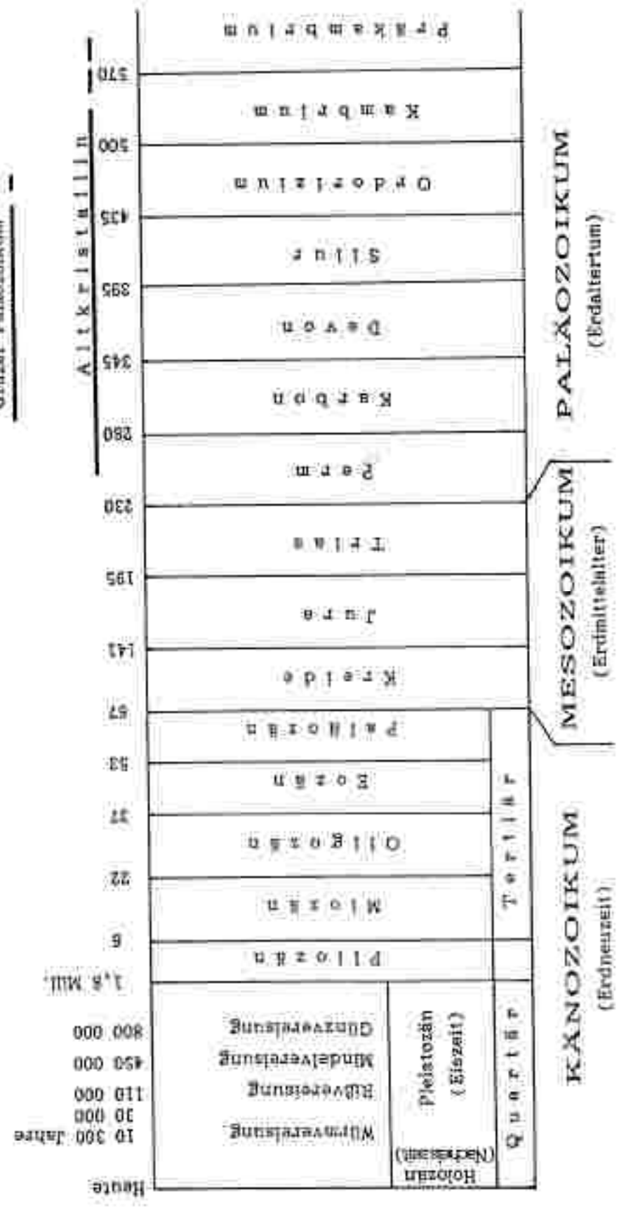
Abb. 1: Straßgraphische Übersicht der geologischen Haupteinheiten im Bezirk Weiz
