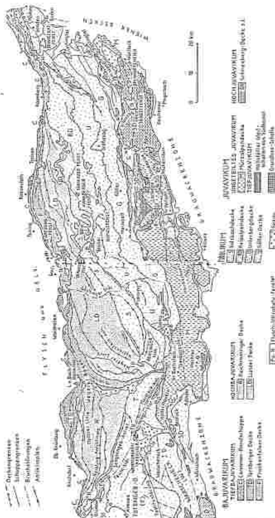
Abb. 5: Tektonische Gliederung der östlichen Kalkalpen (TOLLMANN 1976, LEIN 1981-83 in TOLLMANN 1985)
