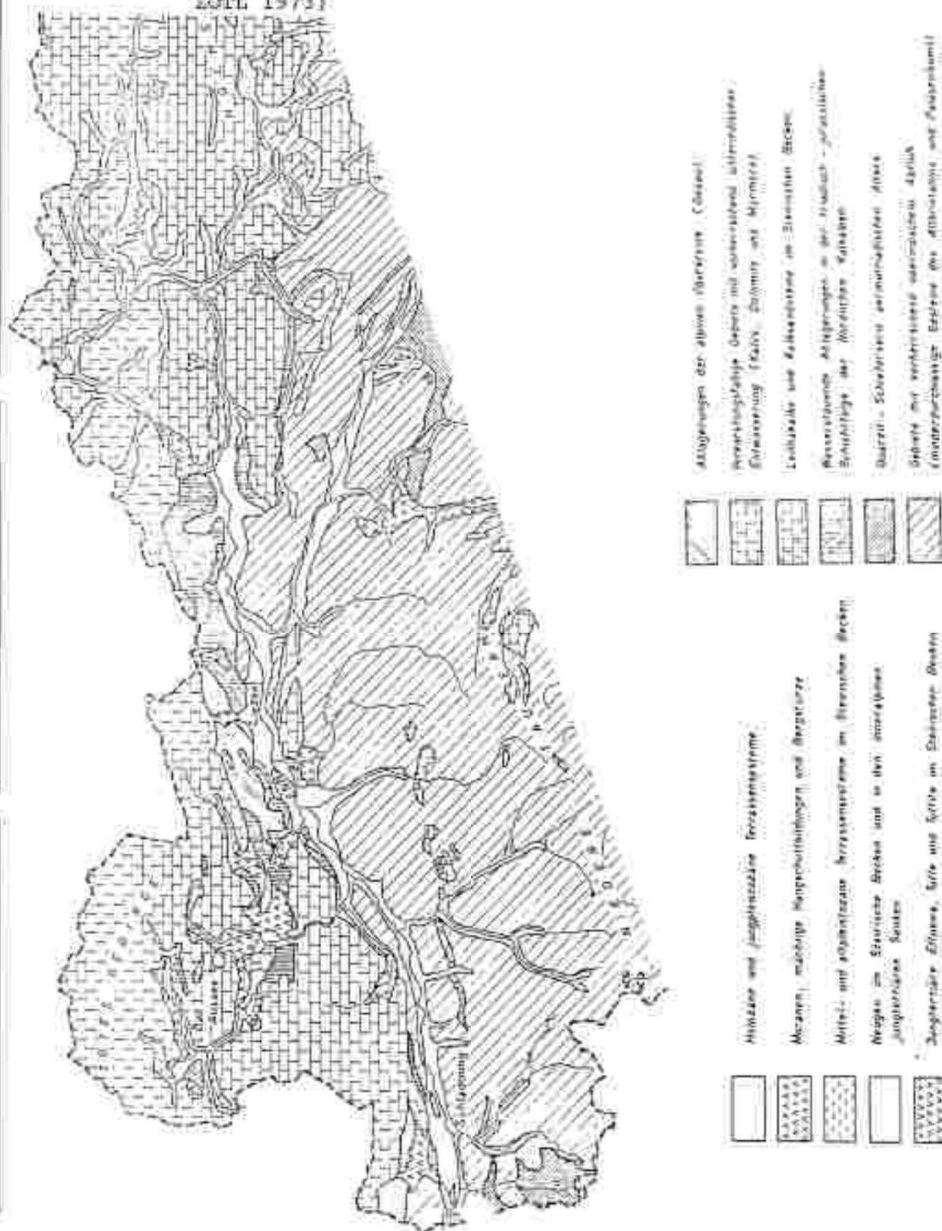
Abb. 43: Die Hydrogeologie des Bezirkes Lienz (Ausschnitt aus EÖTL 1973)
